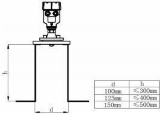
HS83 接管示意图
