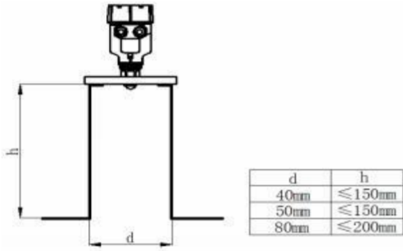
HS80、HS81、HS82 接管示意图
